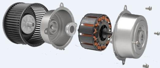
BLDC motor
